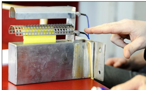
STYR. En temperaturgivare, bilden, och en styrdator är viktiga delar i torkprocessen. Hemligheten är dock programmeringen.
